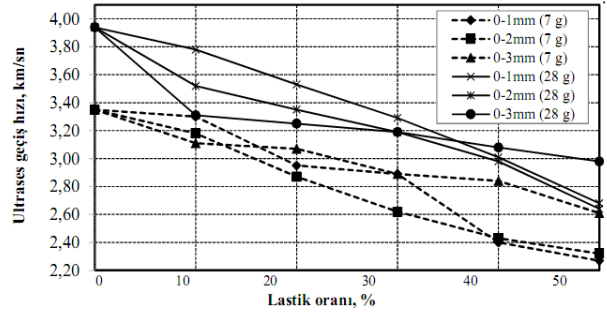
Şekil 4. AOLAHA numunelerinin ultrases geçiş hızları
