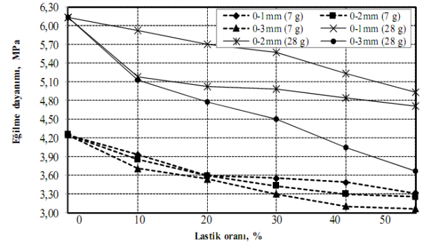
Şekil 5. AOLAHA numunelerinin eğilme dayanımları
