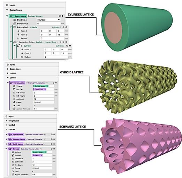
Figure 6. Nerve guide conduits design parameters
