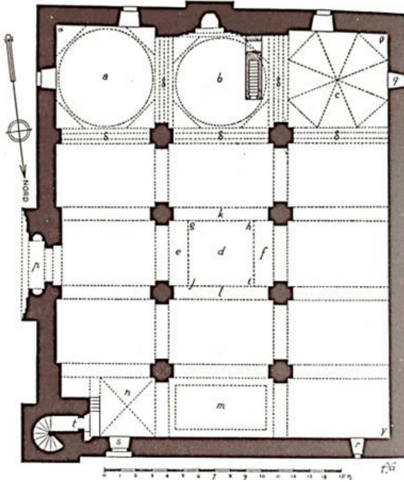
Görsel 14: Niğde Alâeddin Camii planı
