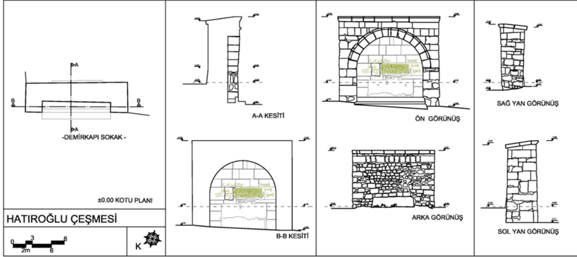
Görsel 16: Hatiroğlu Çeşmesi planı, kesit ve görünüşleri
