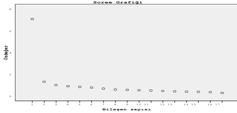
Grafik 1: Özdeğerleri gösteren Scree Grafiği
