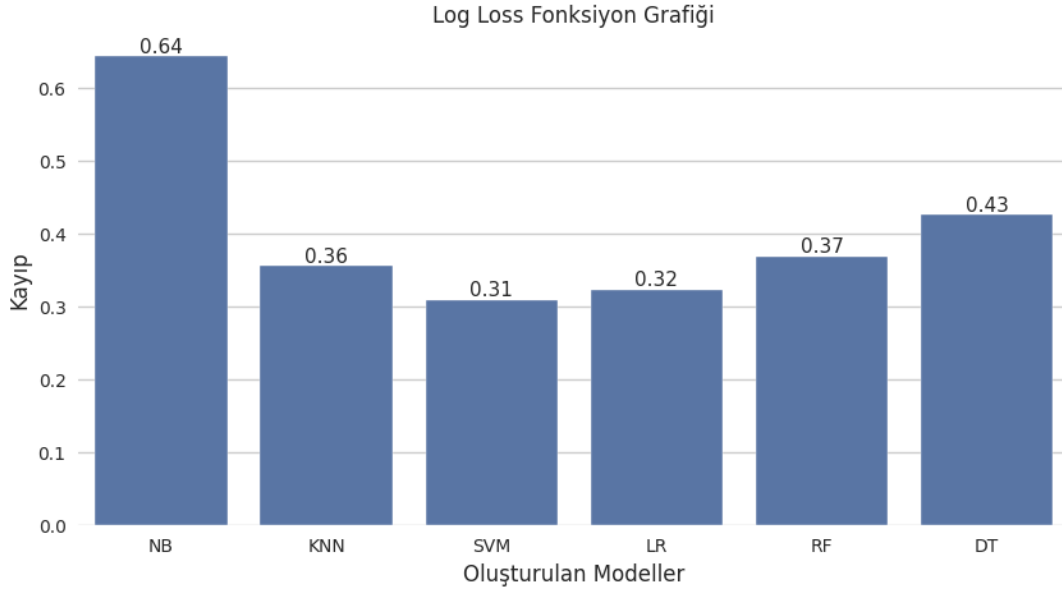
Őekil 7. Log loss fonksiyon grafiđi.
