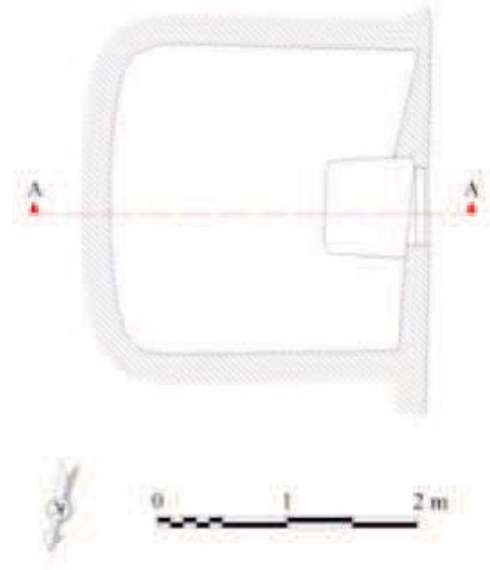
Çizim 1: Yelbeyi Kaya Mezarı Plan ve Kesiti
