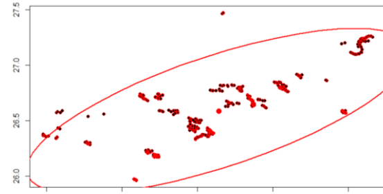
Şekil 8. RES’lere ait standart sapma elipsi
