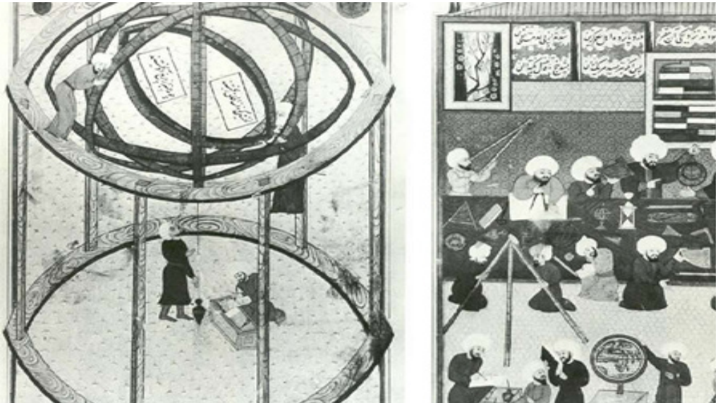
Resim 2: Merâge-Rasathânesi.
