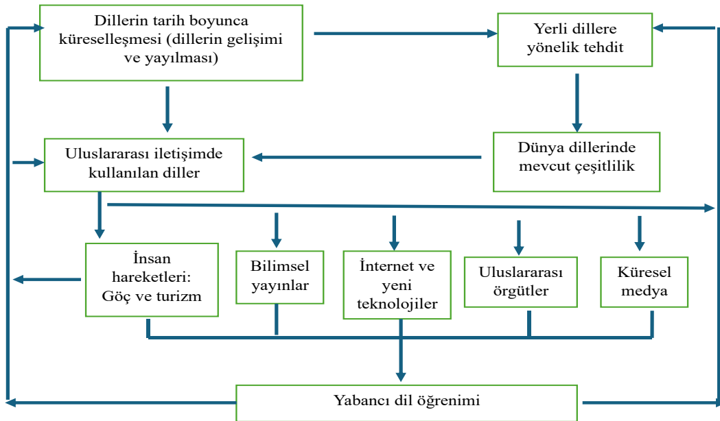
Şekil 1: Dillerin Küreselleşmesi
