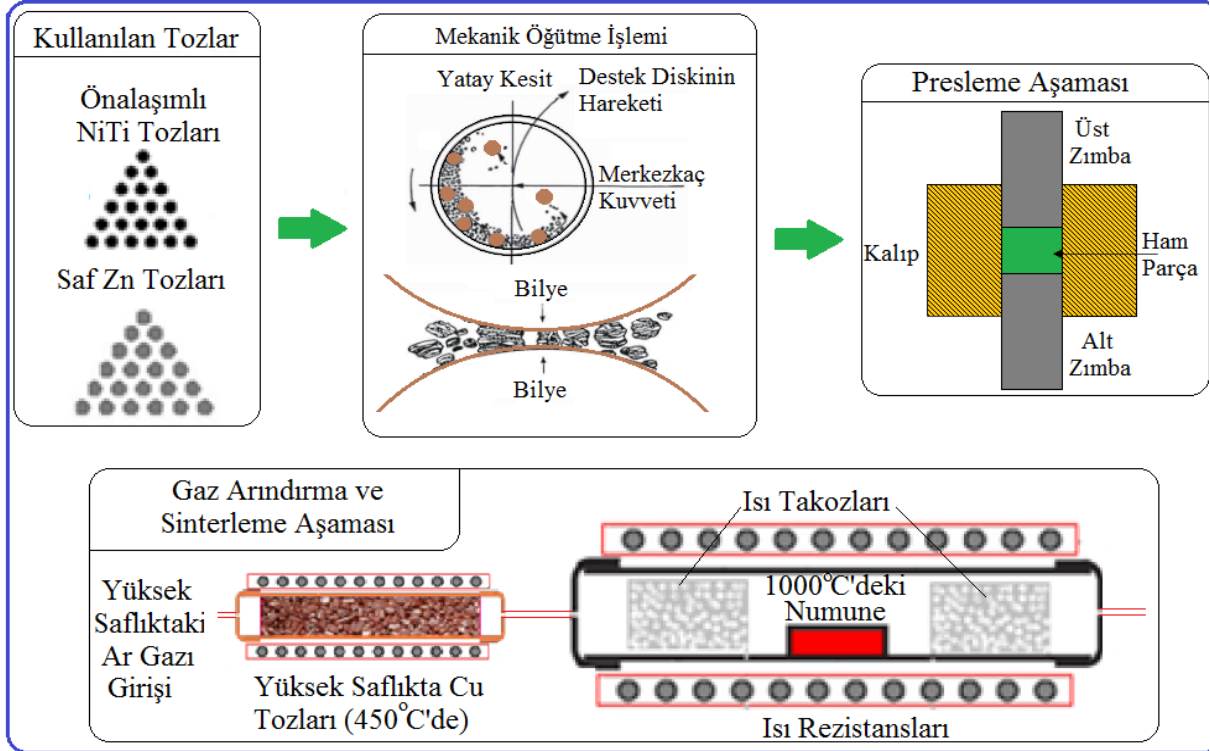
Şekil 3. NiTi - Zn parçalarının üretiminin şematik gösterimi (The schematic diagram about fabrication of NiTi-Zn parts)
