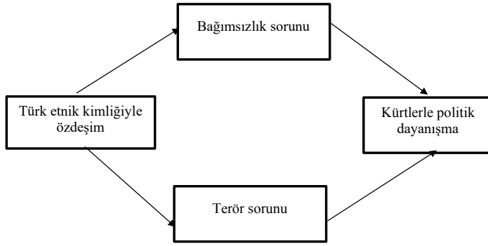
Şekil 1. Birincil grupla politik dayanışma modeli
