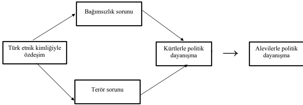
Şekil 2. İkincil grupla politik dayanışma modeli
