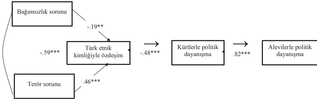
Şekil 4. Yol analizi şeması (Alternatif model)
