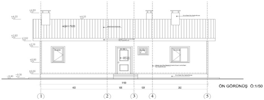
Şekil 4.2 Topaktaş Köyü Köy Ev Ön Görünüşü (TOKİ) [15]
