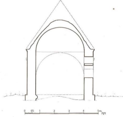
Çizim 4: Anonim Türbe Kesiti ( M.Tunçel'den 2002)
