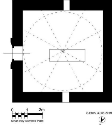
Çizim 1: Sinan Paşa Kümbeti Planı (S. Eren)
