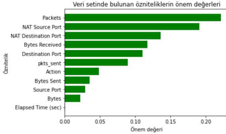
Şekil 4. Veri setinde bulunan özelliklerin önem değerleri
