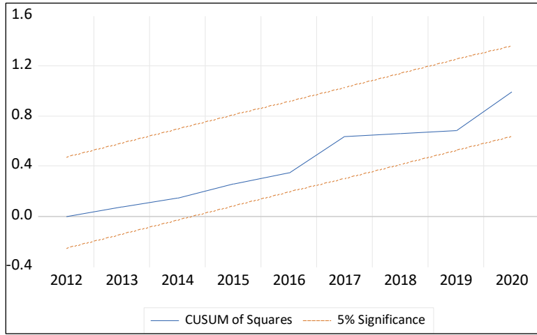
Grafik 1. CUSUM ve CUSUMSQ testi sonuçları
