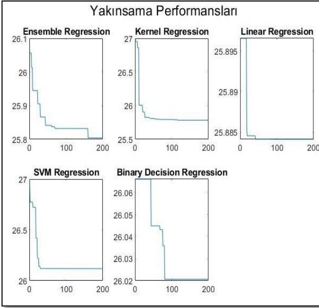
Şekil 3. Yakınsama performansları.
