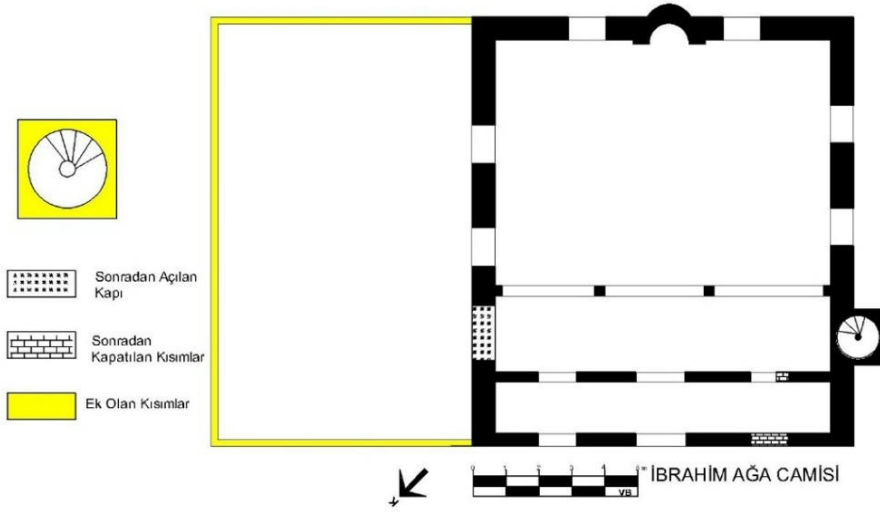
Görsel 20: İbrahim Ağa Camisi Planı (V. Baçaru)
