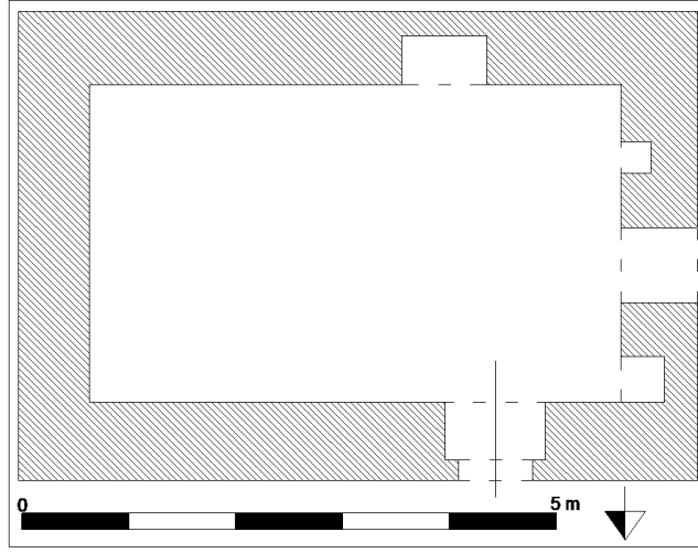
Görsel 23: Kanireş Türbesi Planı
