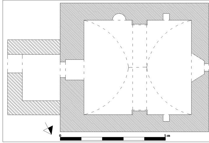
Görsel 4: Şeyhan Türbesi Planı
