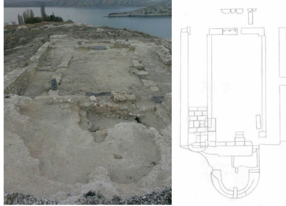
Resim 7. Iuliopolis, 1. No.'lu Bizans Kilisesi, Genel Görünüm ve Rölöve Planı (Sağır, v.d., 2015: 164)
