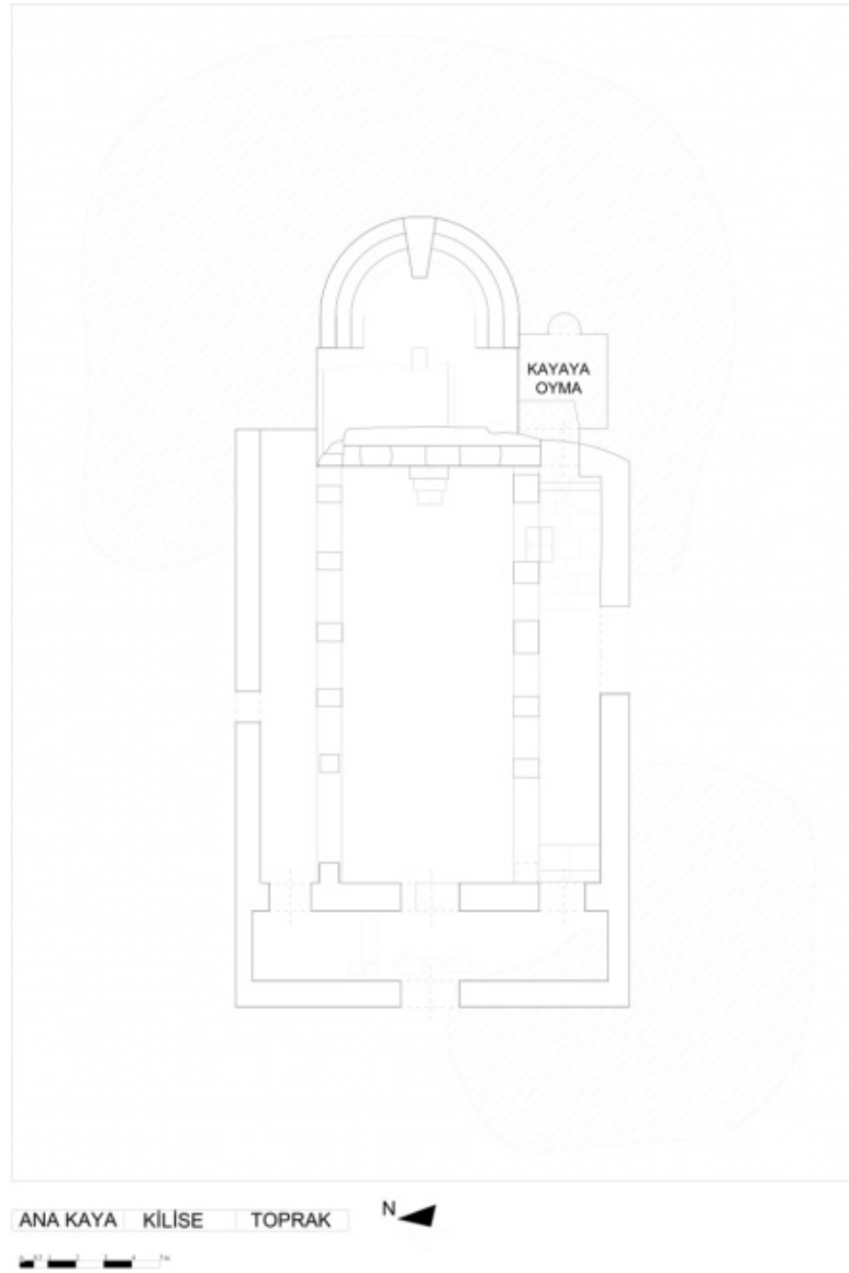
Çizim 1. Iuliopolis, 1 No.'lu Bizans Kilisesi ve Kayaya Oyma Şapel, Rölöve Planı (2024)
