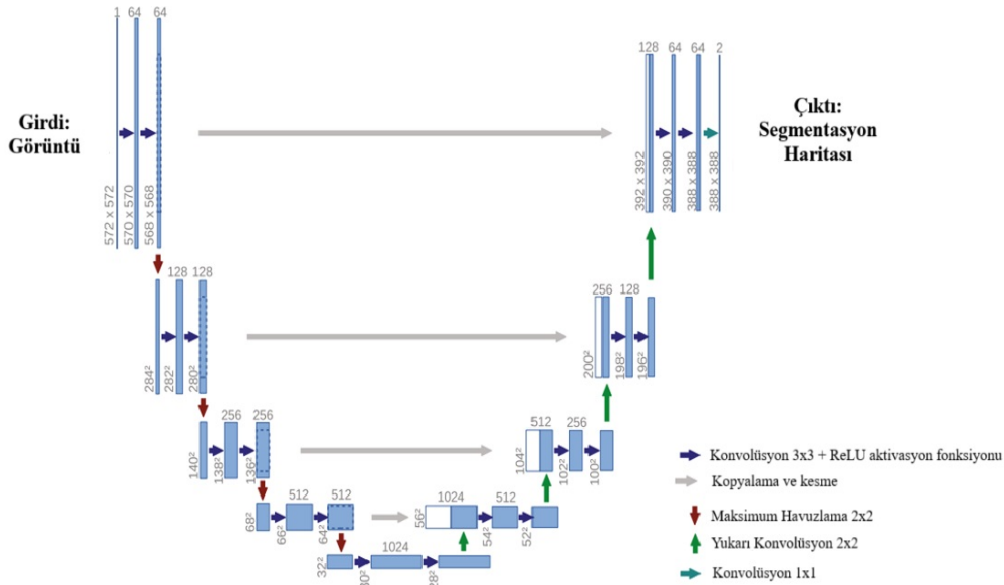
Şekil 4. U-Net mimarisi [25]. (U-Net architecture.)
