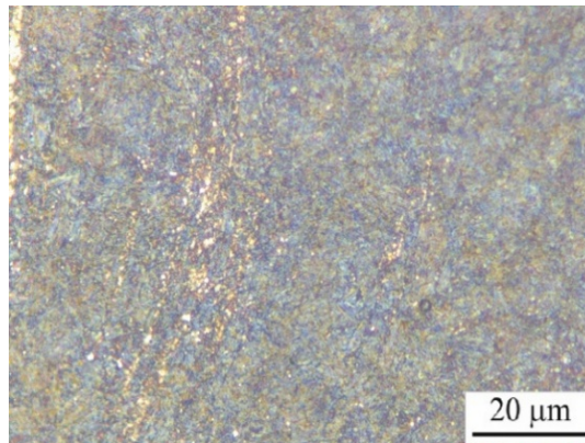
Şekil 6. %2 Nital ve %15 sodyum metabisülfite ile dağlanmış AISI 4340 çeliğinin 1000x büyütmede MM numunesinin martenzitik mikro yapısı. (Optical micrograph of a martensitic microstructure in AISI 4340 steel specimen MM, etched with a solution of 2% Nital and 15% sodium metabisulfite, at 1000x magnification.)
