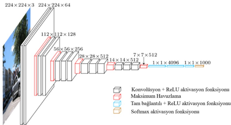
Şekil 3. VGG16 mimarisi [23]. (VGG16 architecture.)
