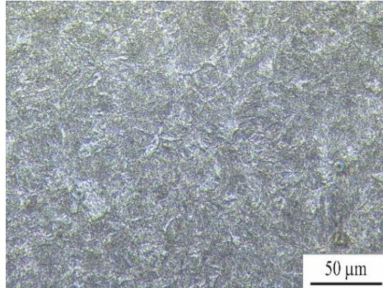
Şekil 7. %2 Nital ile dağlanmış AISI 4340 çeliğinin 500x büyütmede PM numunesinin perlitik mikro yapısı. (Optical micrograph of a pearlitic microstructure in AISI 4340 steel specimen PM, etched with 2% Nital, at 500x magnification.)
