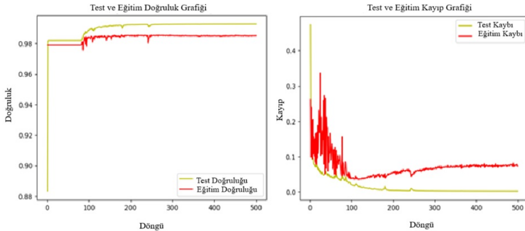
Şekil 10. Kesinlik ve Kayıp grafikleri. (Accuracy and Loss Graphs)
