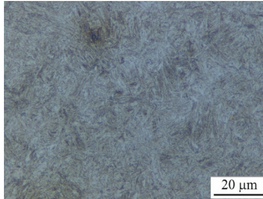
Şekil 5. %2 Nital ile dağlanmış AISI 4340 çeliğinin 1000x büyütmede BM numunesinin optik Beynit mikro yapısı. (Optical microstructure of the BM specimen of AISI 4340 steel etched with 2% Nital at 1000x magnification.)
