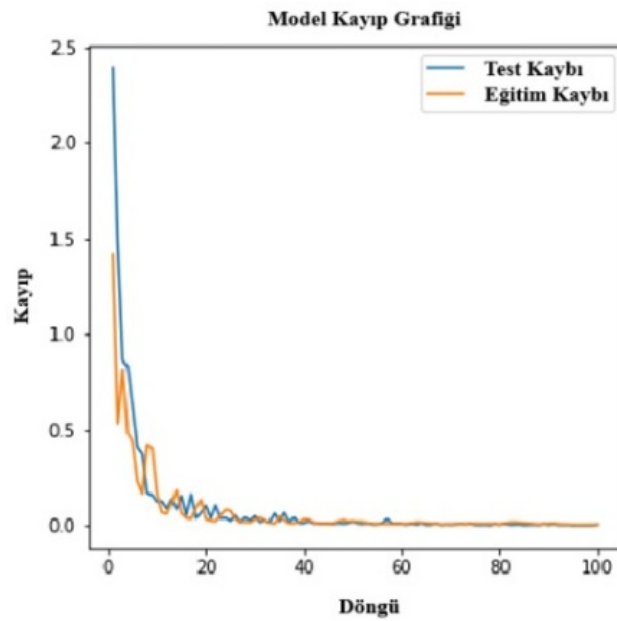
Şekil 8. Kayıp Fonksiyonu. (Loss Function.)
