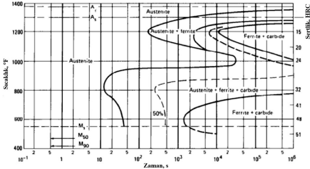
Şekil 2. Farklı mikro yapıların üretilmesinde faydalanılan 4340 çeliğinin izotermal dönüşüm diyagramı [14]. (Isothermal transformation diagram of AISI 4340 steel used for producing different microstructures [14].)
