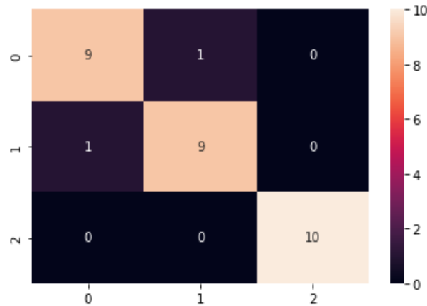
Şekil 9. Karışıklık Matrisi. (Confusion Matrix.)
