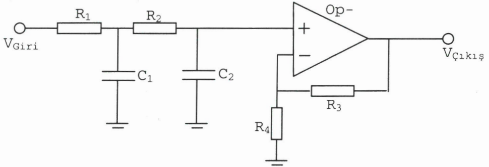
Şekil 4. İkinci dereceden alçak geçiren filtre devresi
