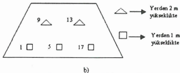
Şekil 2. Yığındaki Isı Sensörlerinin (Pt100) şematik gösterimi, a) Plan, b) AA' kesit.
