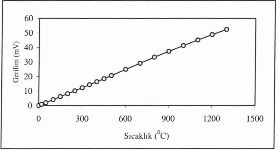
Şekil 3. Pt100'ün Gerilim-Sıcaklık grafiği
