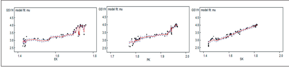
Şekil 8: Model kontrolü
