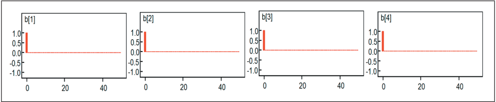
Şekil 7: Otokorelasyon çizimi
