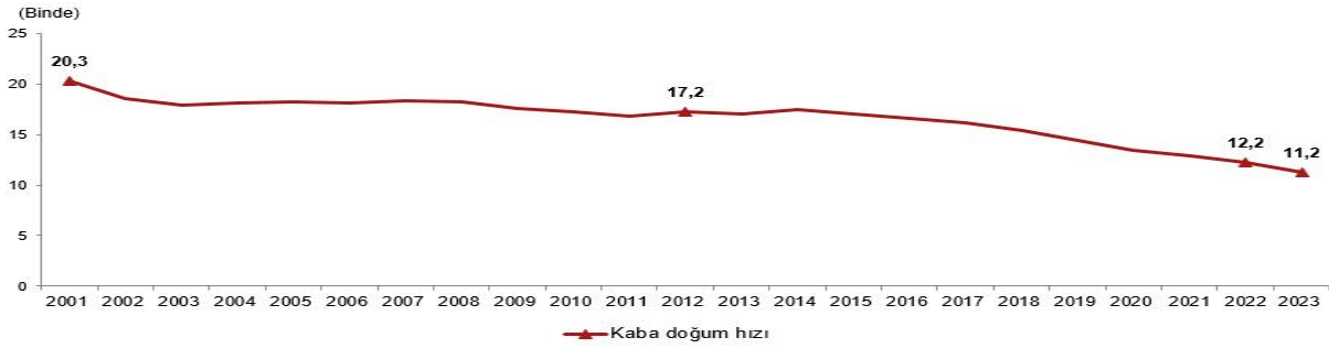
Grafik 2: 2001-2023 yılları arasında Türkiye geneli kaba doğum hızı oranları.
