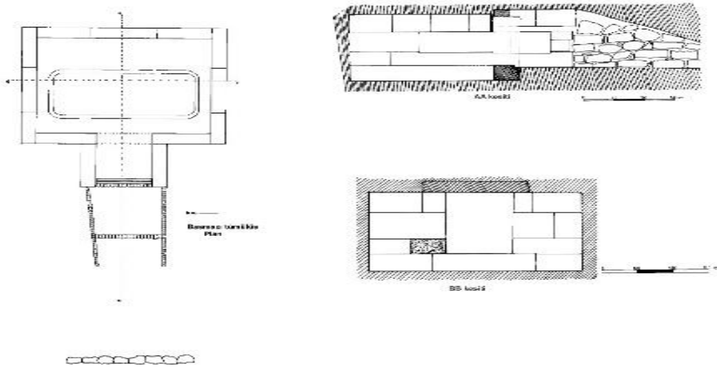
Şekil 3. Basmacı Tümülüsü Plan ve Kesiti (Akbiyikoğlu, 1991: 10-12).
