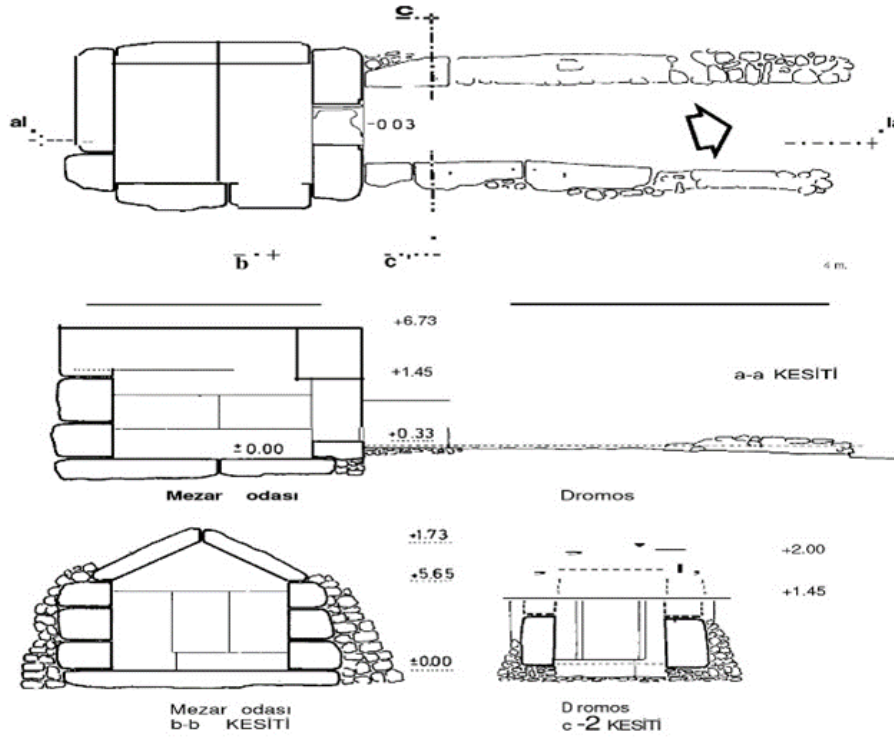
Şekil 12. T1 Tümülü Plan ve Kesiti (İzmirligil, 1975).
