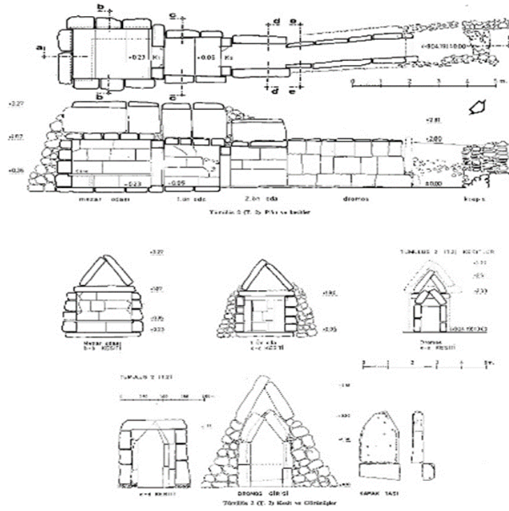
Şekil 14. T2 Tümülüsü Plan ve Kesiti (İzmirligil, 1975).
