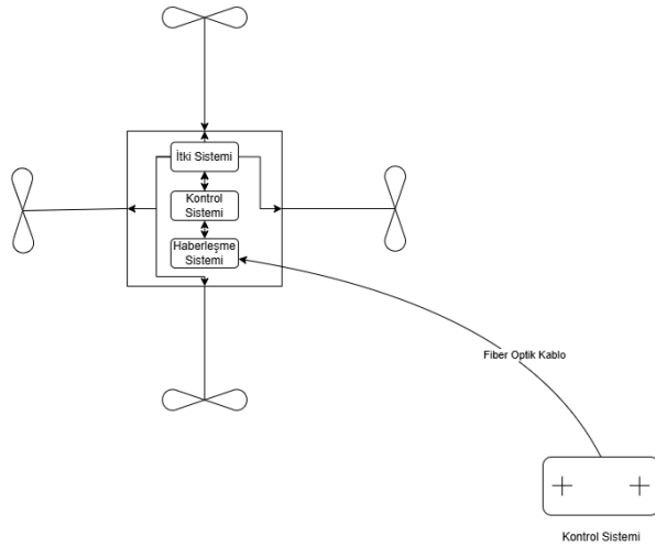
Şekil 3. Kablolu haberleşme sistemine sahip dronun şeması.
