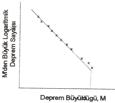
Aşama 2. Deprem büyüklüğü tekrürünün belirlenmesi. Stage 2. Determination of magnitude recurrence.
