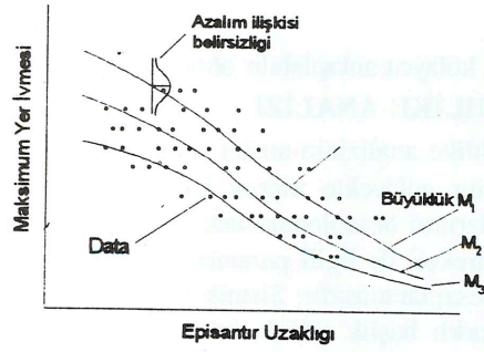
Aşama 3. Azalım ilişkisinin belirlenmesi. Stage 3. Determination of attenuation relationship.
