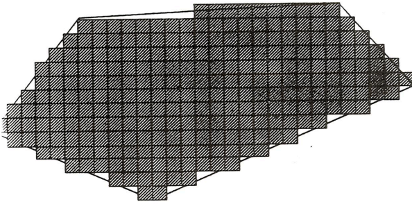
Şekil 9. Poligon (üçgen, beşgen, vs) şeklinde tanımlanan sismik kaynağın orjinal sınırları ile sismik kaynak için tutulmuş olan hücrelerin karşılaştırmalı olarak gösterimi.
