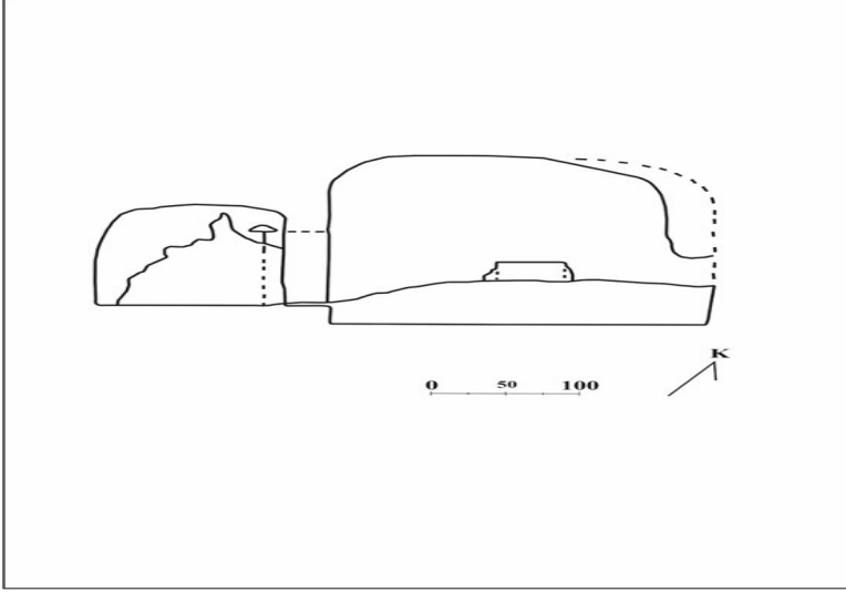
Görsel 4. Çetintaş (Hergel) Kaya Mezarının Planı AA Kesiti
