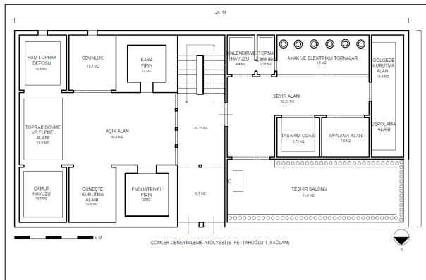
Görsel 8. Günümüz İçin Önerilen Çömlek Üretim Atölyesi Plan Denemesi ve Trabzon'da Çömlekçi Dükkanı (M. Reşat Sümerkan Kişisel Arşivi)
