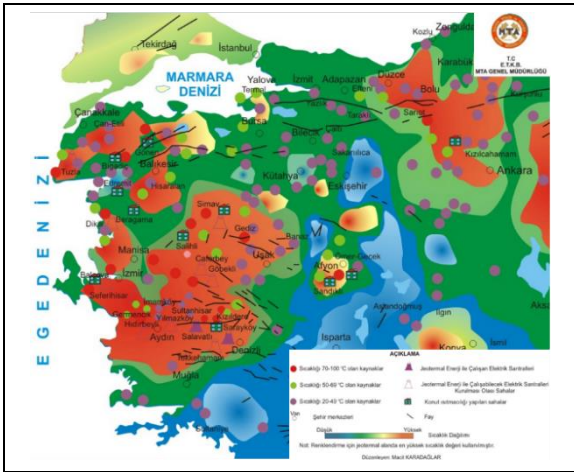
Şekil 5. Denizli jeotermal kaynak potansiyeli.
