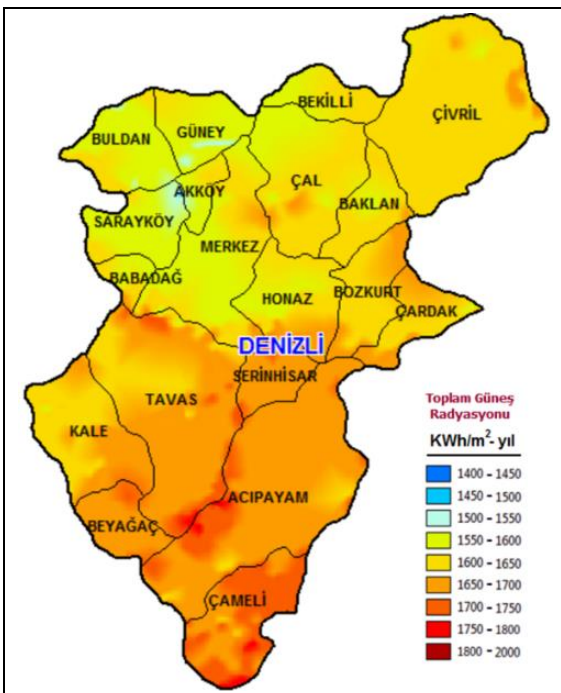
Şekil 6. Denizli güneş enerjisi potansiyeli atlası.
