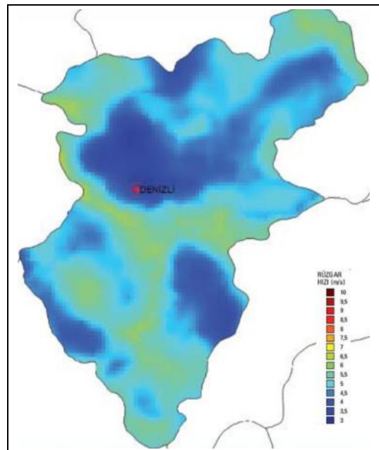
Şekil 7. Denizli rüzgar hızı dağılımı - 50 m.
