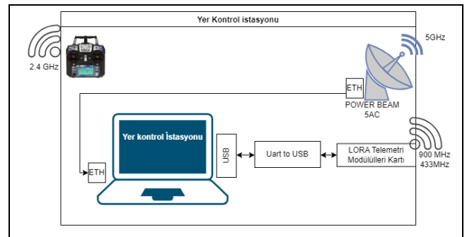
Şekil 8. Yer kontrol istasyonu mimarisi.
