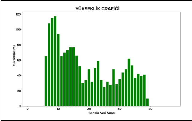
Şekil 13. İHA'dan alınan yükseklik verisi.
