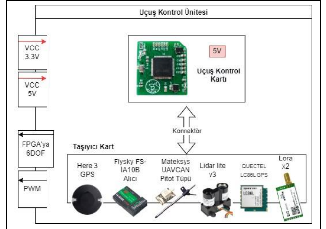
Şekil 3. Uçuş kontrol ünitesi.
