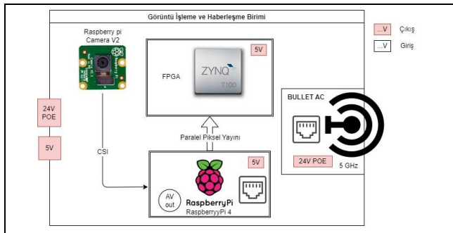
Şekil 7. Görüntü işleme ve haberleşme birimi.
