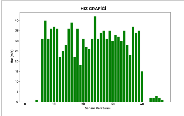
Şekil 15. İHA'dan alınan hız verisi.
