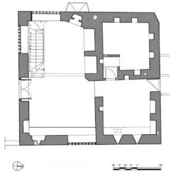
Şekil 12: Safranbolu, Kıranköy, Saffronia 1900 Konak Otel, zemin kat planı
