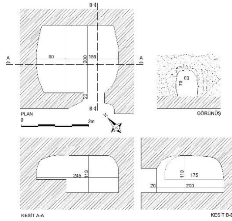
Fig. 4c: KM3 plan, kesit ve görünüş çizimi
