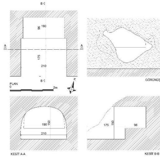
Fig. 13b: KM18 plan, kesit ve görünüş çizimi.
