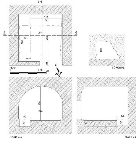
Fig. 9c: KM10 plan, kesit ve görünüş çizimi.
