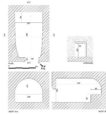
Fig. 3c: KM2 plan, kesit ve görünüş
