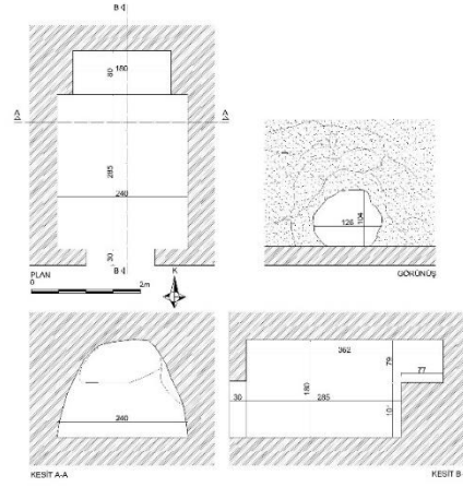
Fig. 12c: KM17 plan, kesit ve görünüş çizimi.
