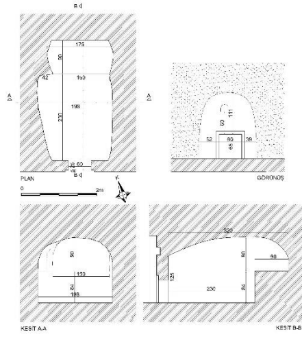
Fig. 8c: KM7 plan, kesit ve görünüş çizimi.
