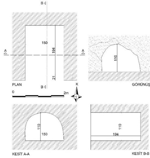
Fig. 11b: KM15 plan, kesit ve görünüş çizimi.
