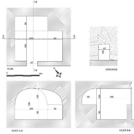
Fig. 10c: KM14 plan, kesit ve görünüş çizimi.
