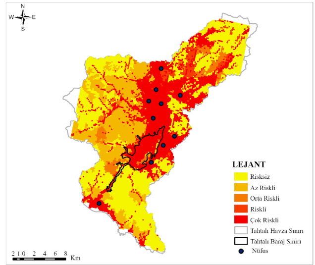
Şekil 5. Tahtalı Barajı Havzası Taşkın Risk Haritası
