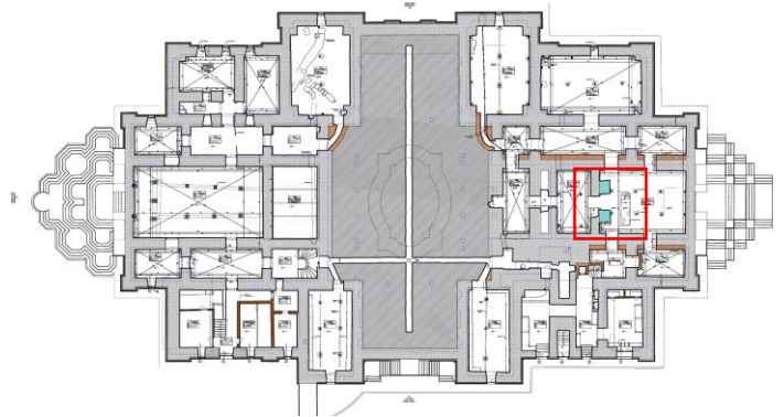
Şekil 16. Bodrum Kata Sonradan Eklenen Kâgir Ayaklar (Bodrum kat planı, Hanart Mimarlık, 2022)
