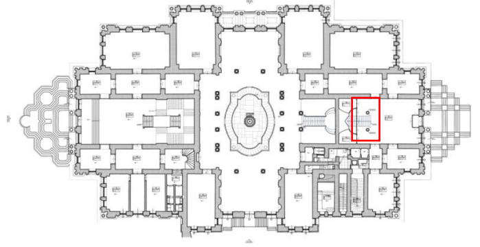
Şekil 14. Zemin Kata Sonradan Eklenen Ahşap Sütunlar (Zemin kat planı, Hanart Mimarlık, 2022)
