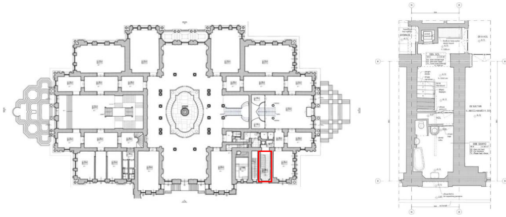
Şekil 8. II. Abdülhamid'e Ait Banyonun Planı (Zemin kat rölöve planı, Hanart Mimarlık, 2022)
