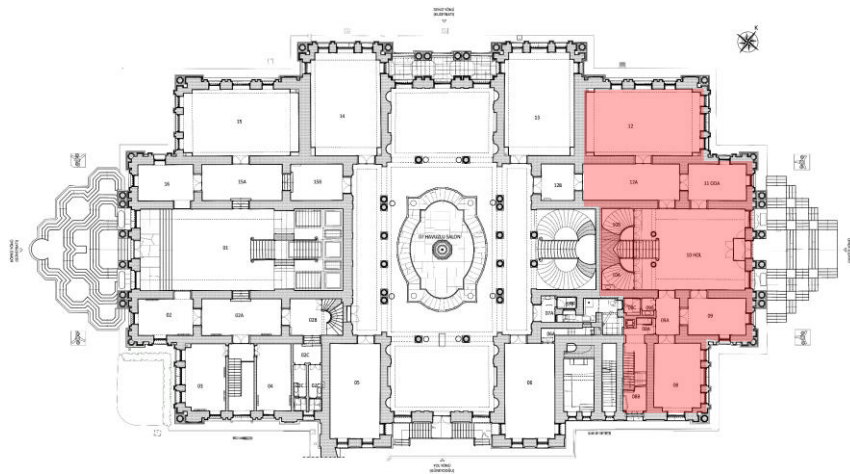
Şekil 7. Sarayda II. Abdülhamid'in Kullanımı İçin Ayrılan Harem Dairesi (Zemin Kat planı, Hanart Mimarlık, 2022)
