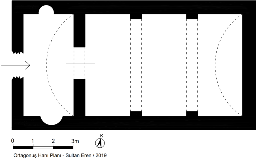
Levha 1: Ortagonuş Hanı Plan
