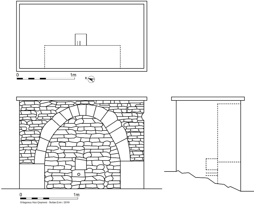
Levha 2: Ortagonuş Han Çeşmesi planı ve Cephe Görünüşü
