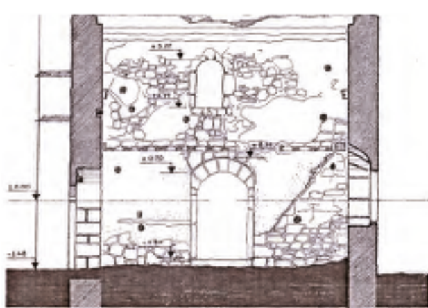
Res. 7 - Kilise D-D kesiti.
