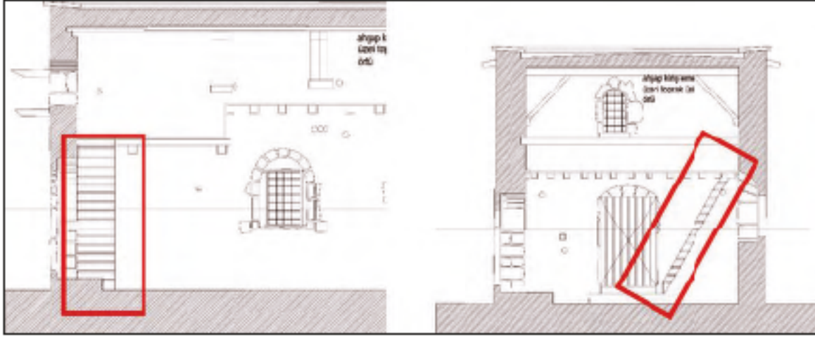
Res. 17 - Restitüsyon önerisi, AA ve CC kesiti.
