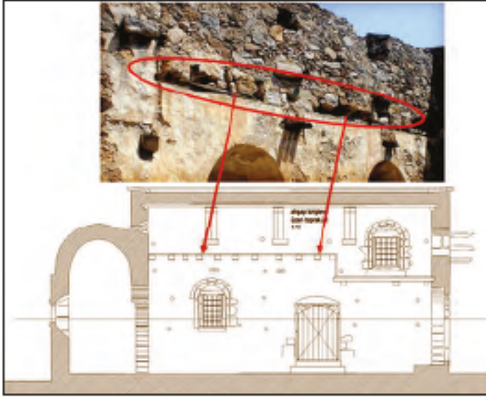
Res. 13 - Restitüsyon önerisi, B-B kesiti.
