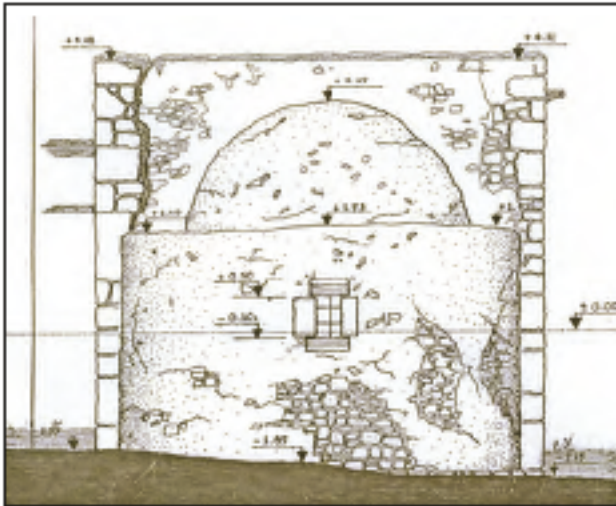
Res. 11 - Kilise batı cephesi.
