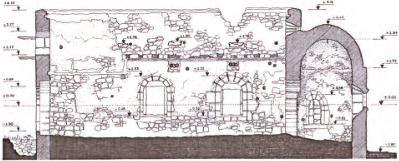
Res. 5 - Kilise B-B kesiti.
