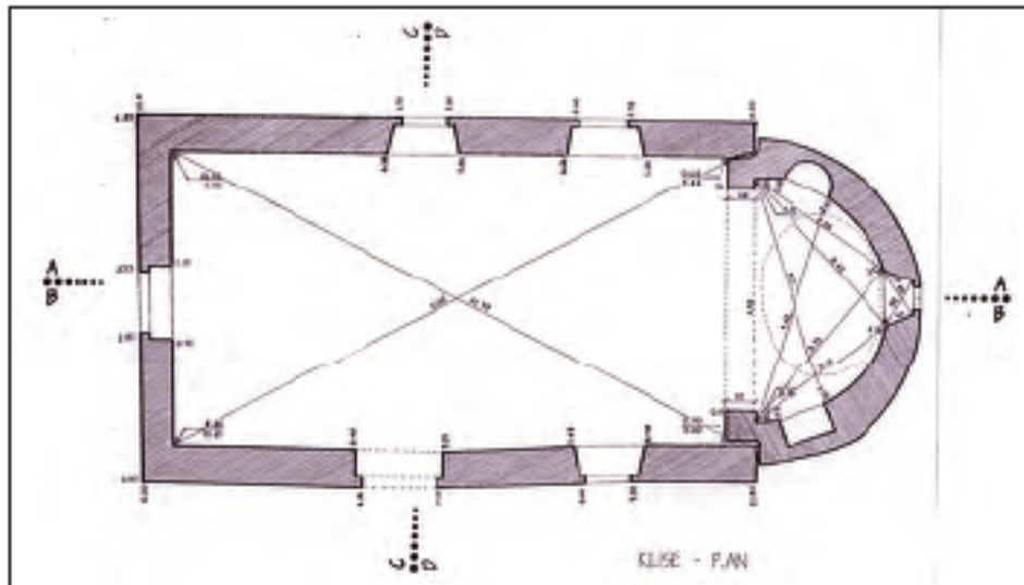
Res. 3 - Kilise durum planı.
