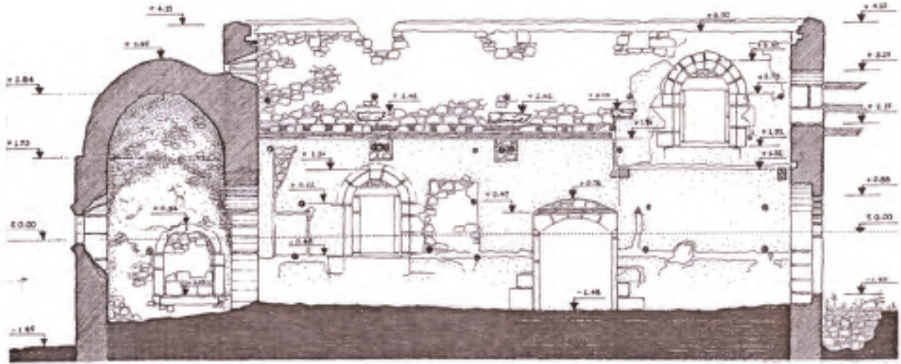
Res. 6 - Kilise C-C kesiti.
