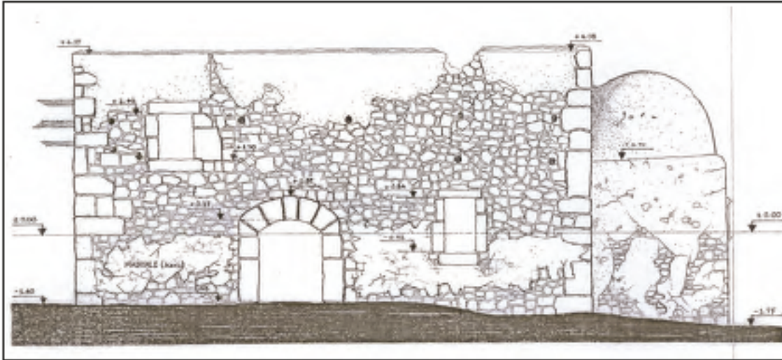
Res. 10 - Kilise doğu cephesi.
