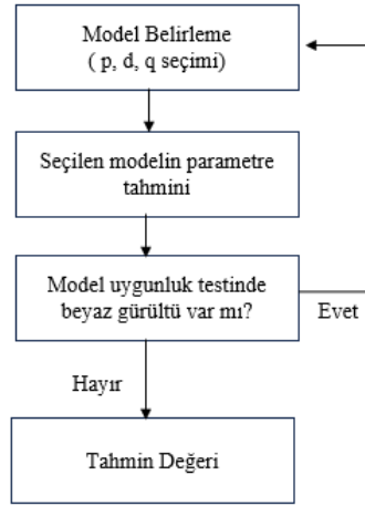
Şekil 3: Model Kurma Aşamaları (Box ve Jenkins 1976)
