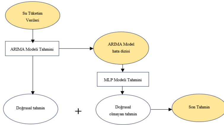
Şekil 4: Hibrit ARIMA-MLP Tahmin Modeli Akış Şeması
