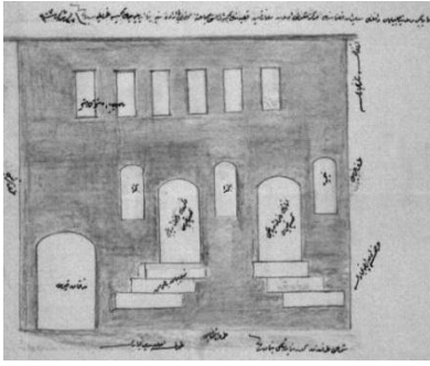
Kilisenin Kuzey ve Batı Cephesi.
