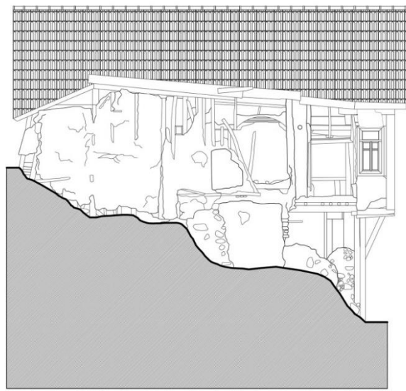
Sol Yan Görünüş Ölçek: 1/50
