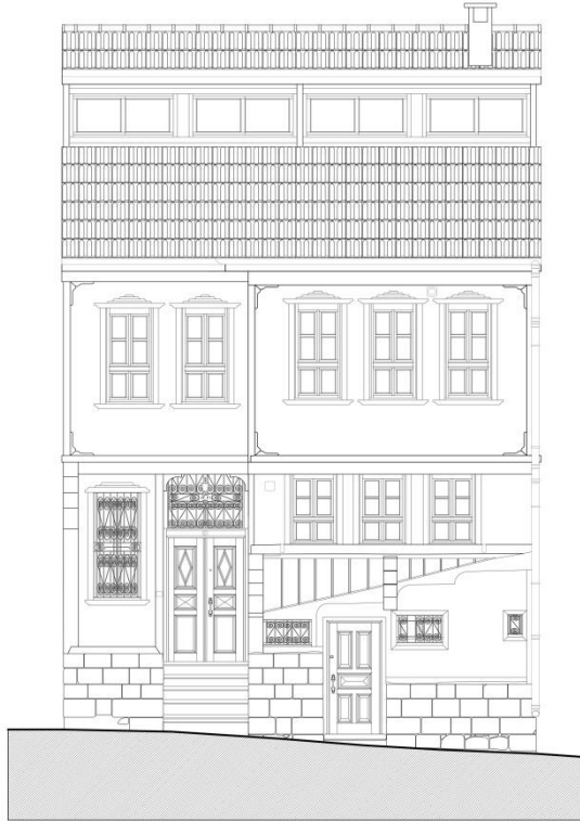
Ön Görünüş Ölçek: 1/50 Çizim: Kadir Deniz
