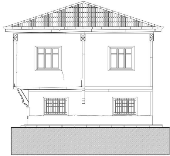
Sağ Yan Görünüş Ölçek: 1/50
