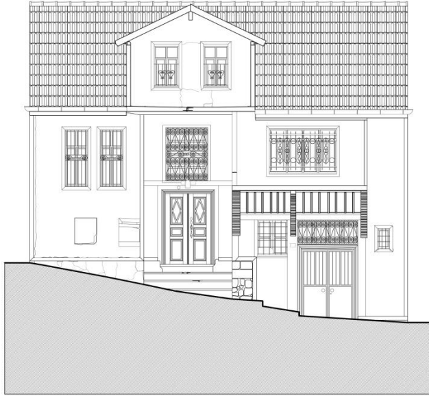
Ön Görünüş Ölçek: 1/50 Çizim: Kadir Deniz
