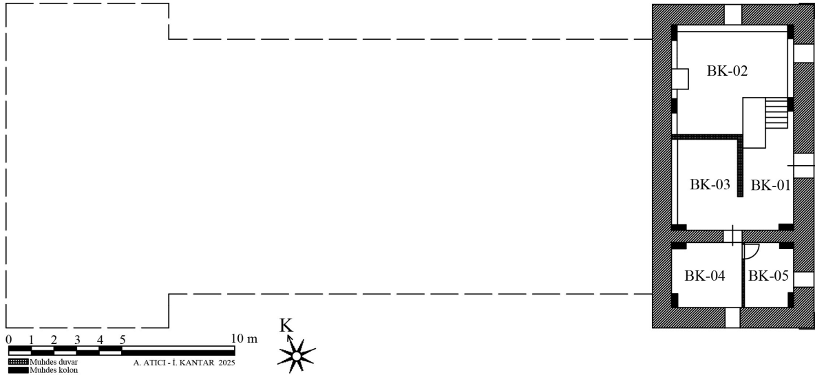
Şekil 20. Gerze İnkılap Yatı Mektebi'nin bodrum kat planı.
