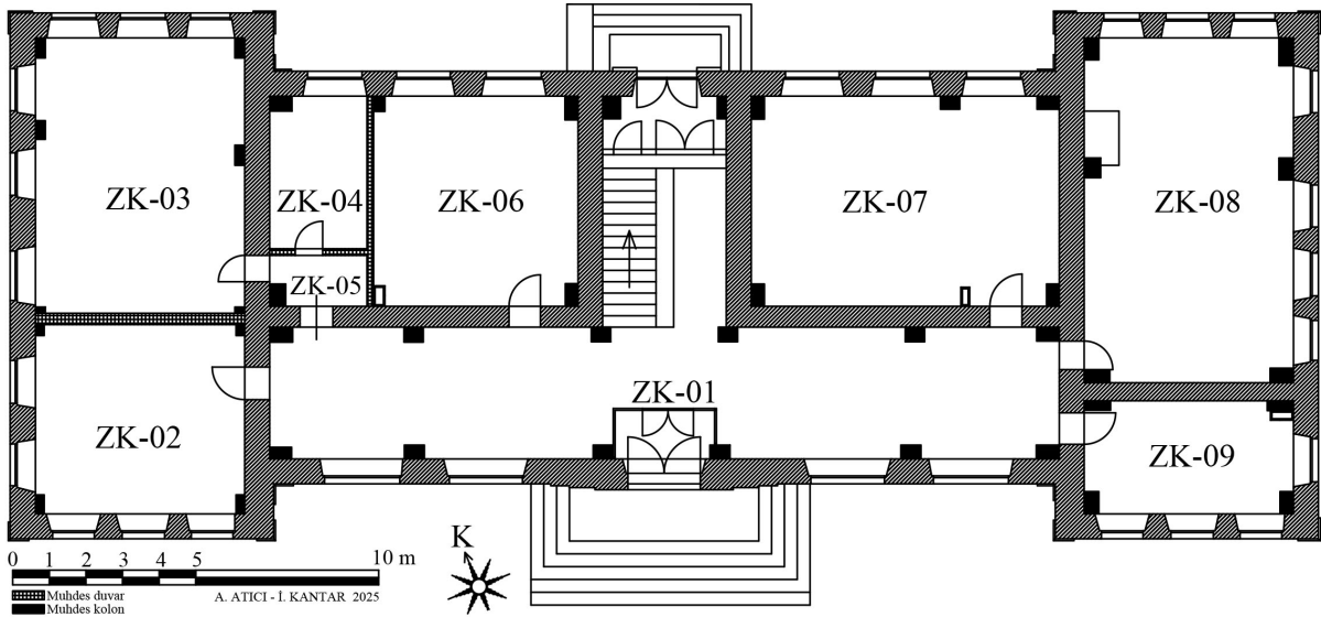
Şekil 28. Gerze İnkılap Yatı Mektebi'nin zemin kat planı.
