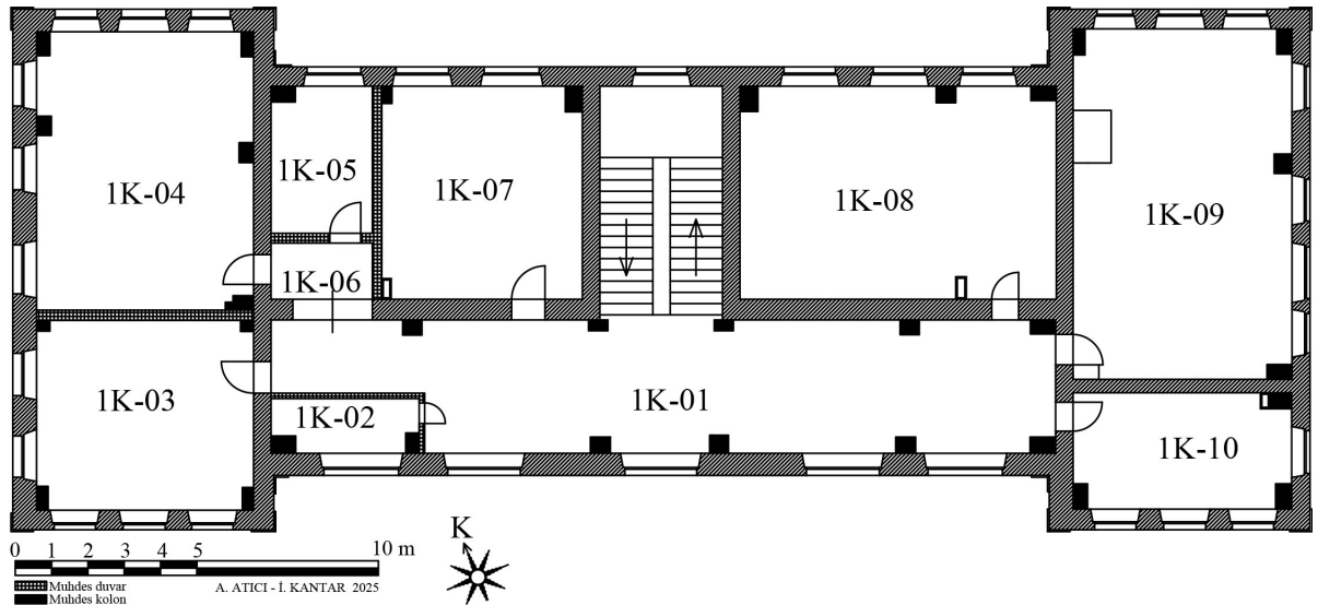
Şekil 31. Gerze İnkılap Yatı Mektebi'nin birinci kat planı.
