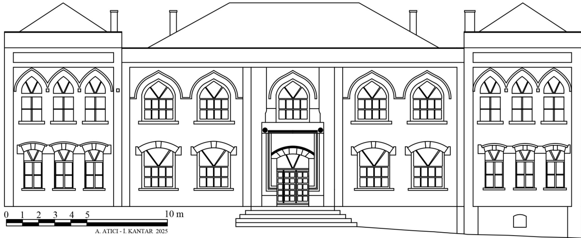
Şekil 19. Gerze İnkılap Yatı Mektebi'nin güney cephe çizimi.
