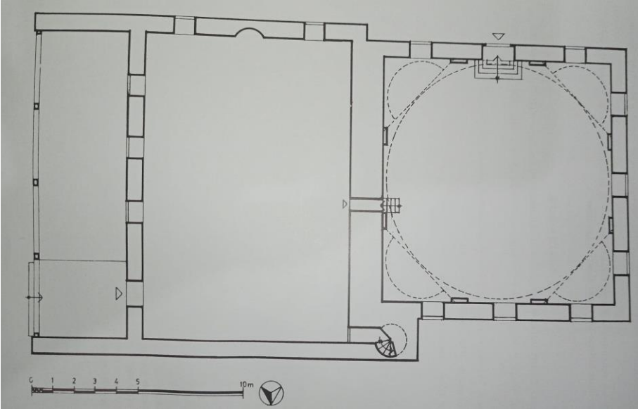
Plan 1. Emirci Sultan Cami ve Türbesi'nin planı 70
