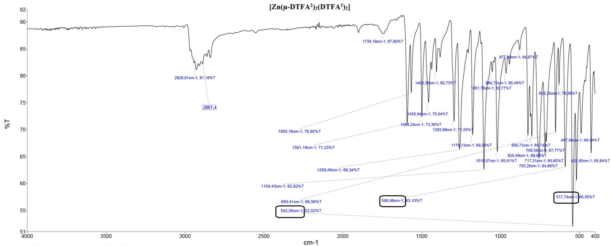
Scheme 2b. IR spectrum of [Zn( \mu -DTFA 2 ) 2 (DTFA 2 ) 2 ] (4000-400 cm -1 ).
