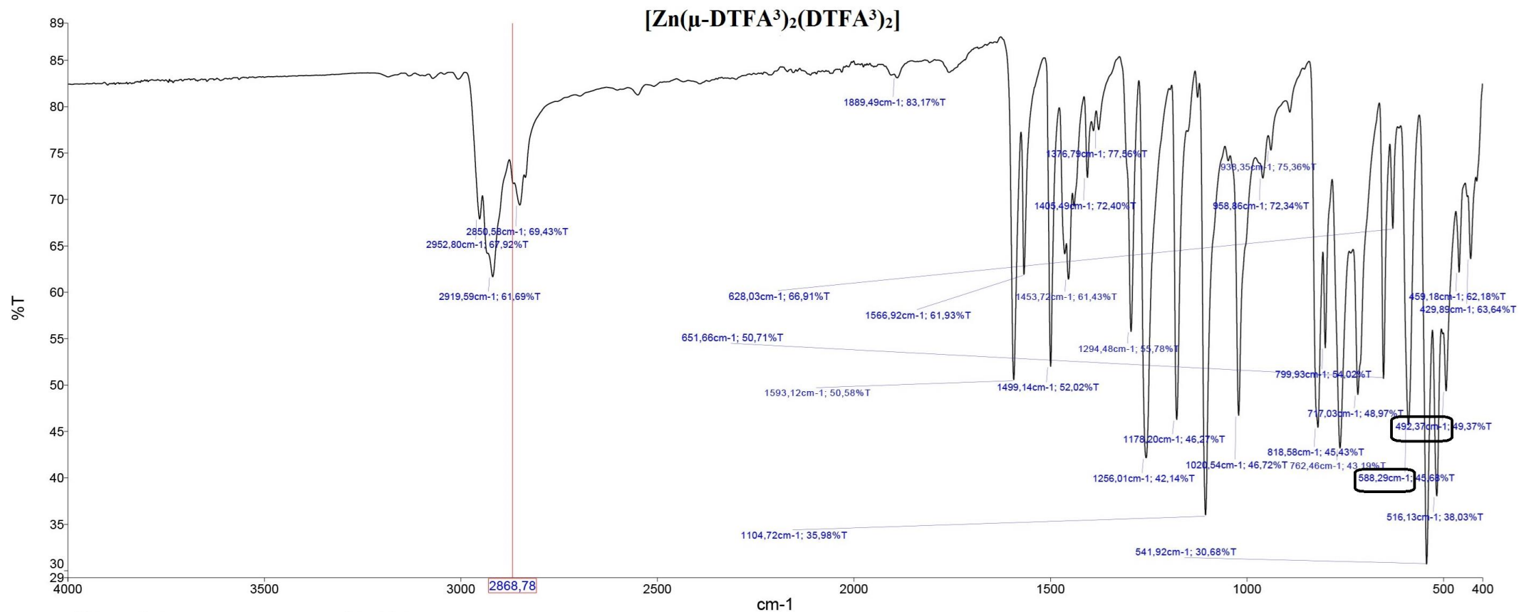
Scheme 3b. IR spectrum of [Zn( \mu -DTFA 3 ) 2 (DTFA 3 ) 2 ] (4000-400 cm -1 ).
