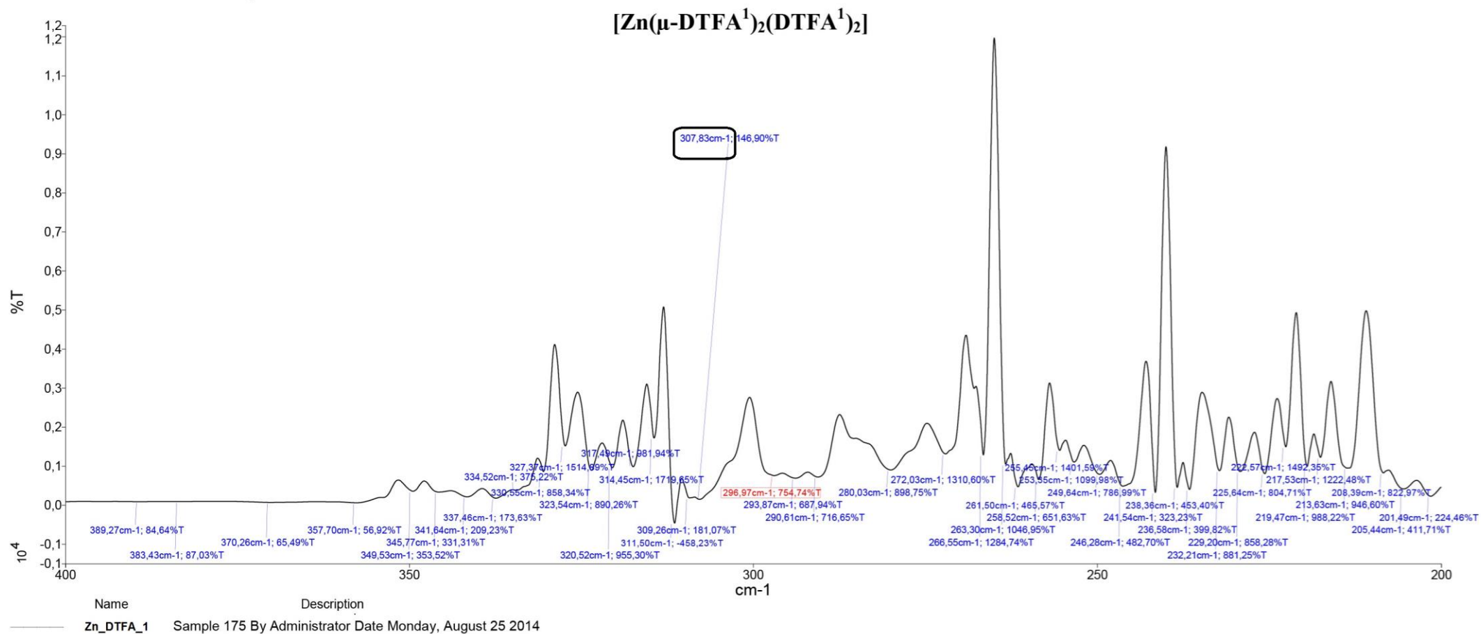
Scheme 1a. IR spectrum of [Zn( \mu -DTFA 1 ) 2 (DTFA 1 ) 2 ] (400-200 cm -1 ).
