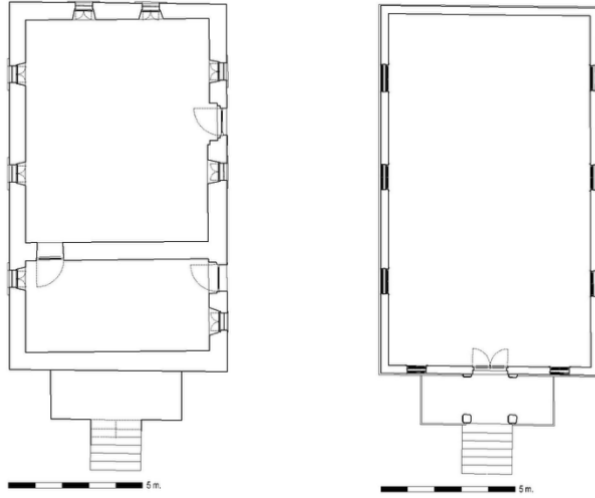
Çizim 1-2: Kilisenin Alt ve Üst Kat Planı.
