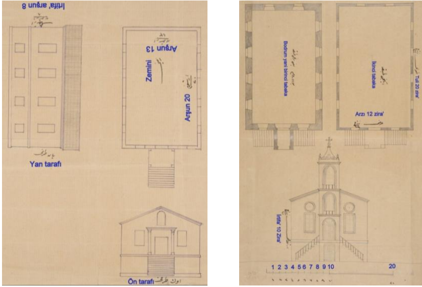
Çizim 3-4: Zincidere’de İnşa Edilecek Kilise İçin Hazırlanan Tasarım Örnekleri (BOA, İ. AZN, 1-5/1, 2).
