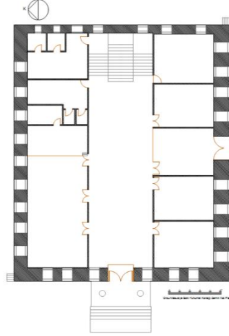
Çizim 1. Ordu/Mesudiye Eski Hükümet Konağı Zemin Kat Planı
