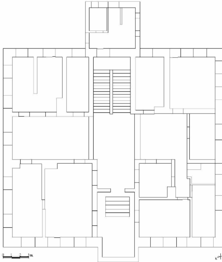
Görsel 28. Bergama Hükümet Konağı Zemin Kat Planı (R Toptaş'tan)
