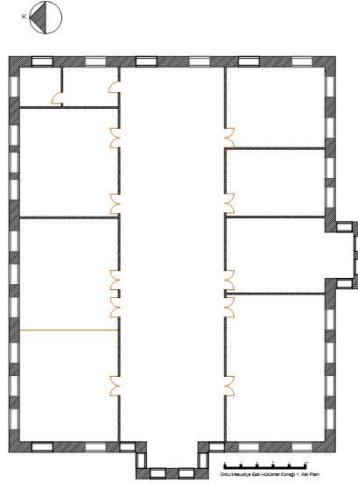
Çizim 2. Ordu/Mesudiye Eski Hükümet Konağı 1. Kat Planı
