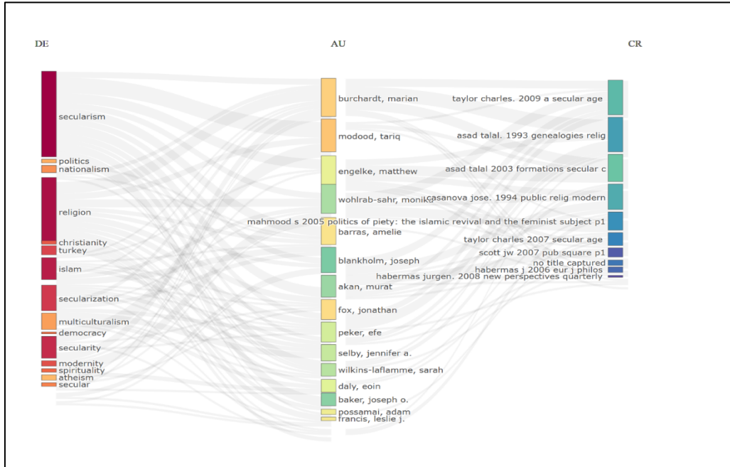
Şekil 19: Kelime-Yazar-Atıf ilişkileri
