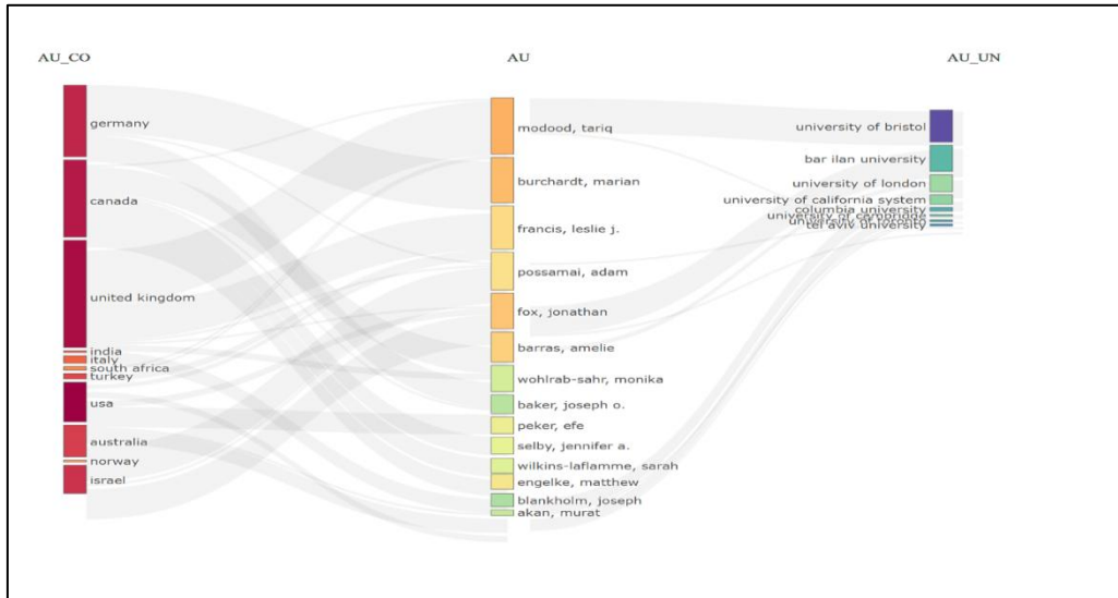
Şekil 17: Ülke-Yazar-Kurum İlişkileri
