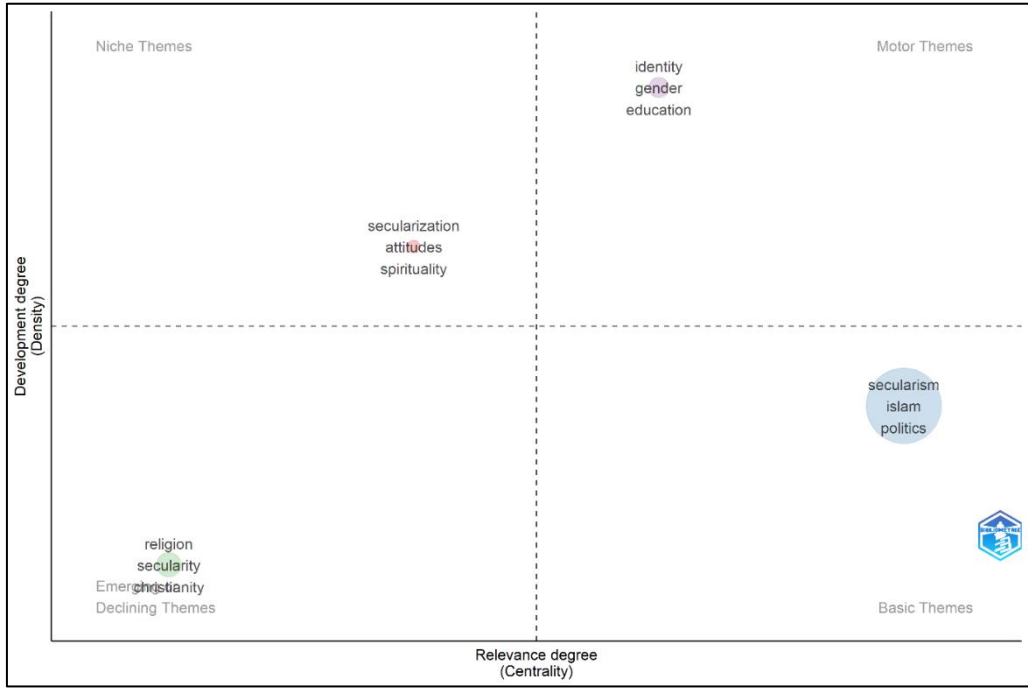
Şekil 15: Tematik Haritalama
