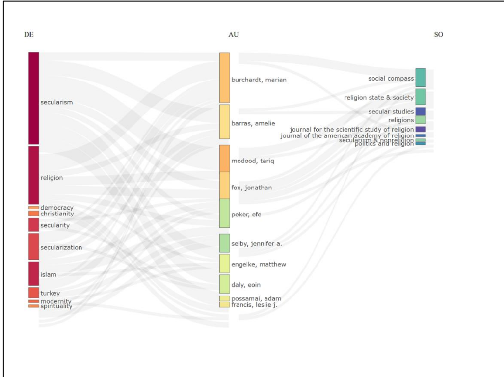
Şekil 18: Kelime-Yazar-Dergi İlişkileri
