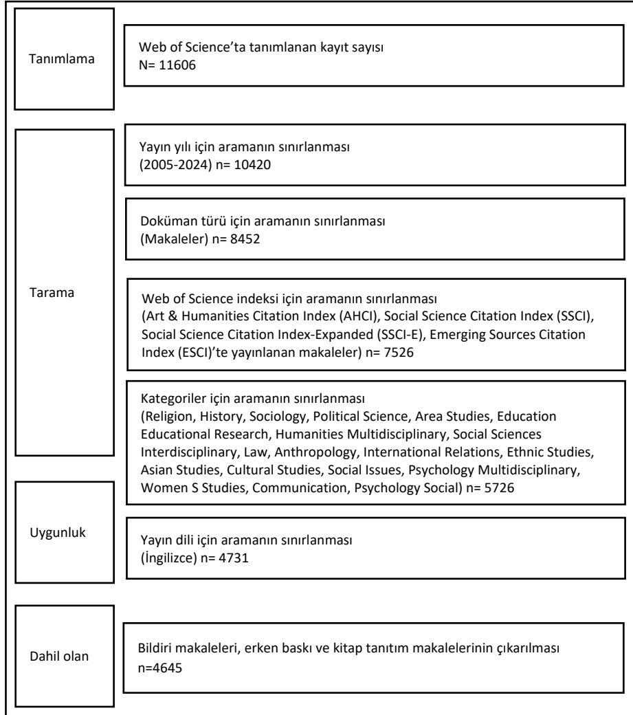
Şekil 1: PRISMA şeması
