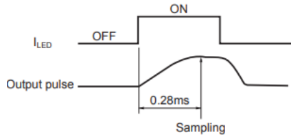
Şekil 4. Çıkış Darbesinin Örnekleme Zamanı
