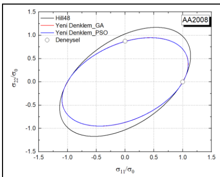
Şekil 4. AA2008 alaşımında akma yüzeylerinin karşılaştırması.
