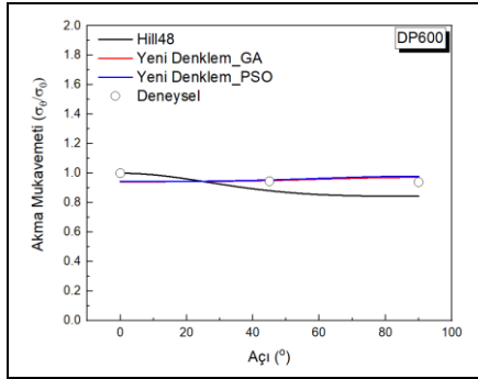
Şekil 2. DP600 çeliğinde akma gerilmesi oranının açıyla değişimi.
