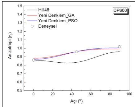
Şekil 3. DP600 çeliğinde anizotropinin açıyla değişimi.
