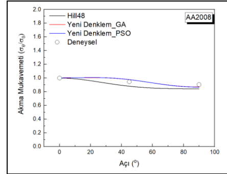
Şekil 5. AA2008 alaşımında akma gerilmesi oranının açıyla değişimi.
