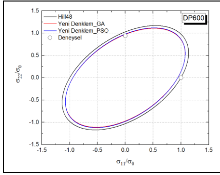
Şekil 1. DP600 çeliğinde akma yüzeylerinin karşılaştırması.
