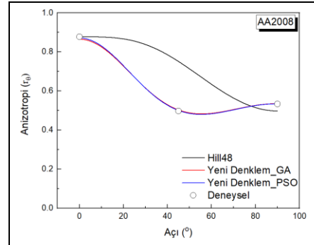
Şekil 6. AA2008 alaşımında anizotropinin açıyla değişimi.
