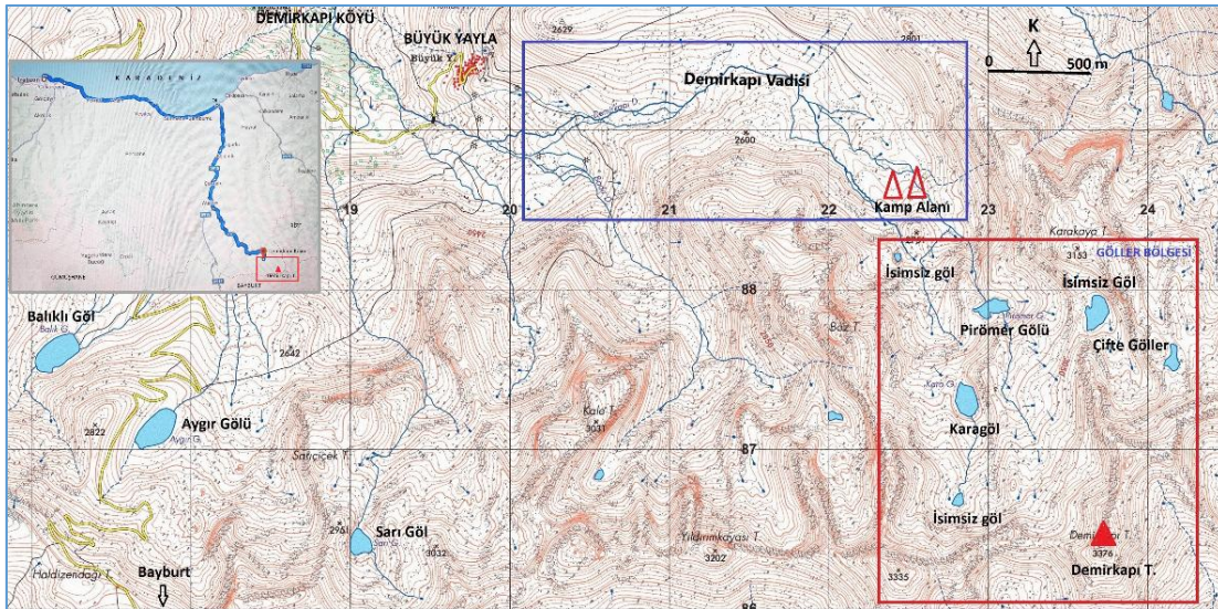
Şekil-1 Demirkapı vadisi, buzul gölleri ve Demirkapı zirvesinin konum haritası
