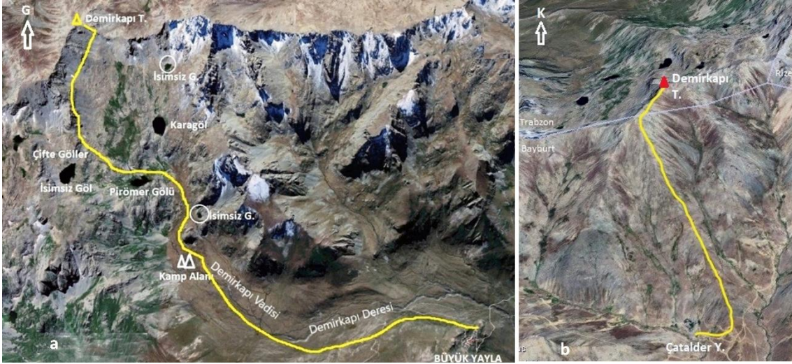
Şekil-5 Demirkapı zirvesi (a) kuzey, (b) güney yamacı tırmanma rotaları ve buzul gölleri (Google Earth)
