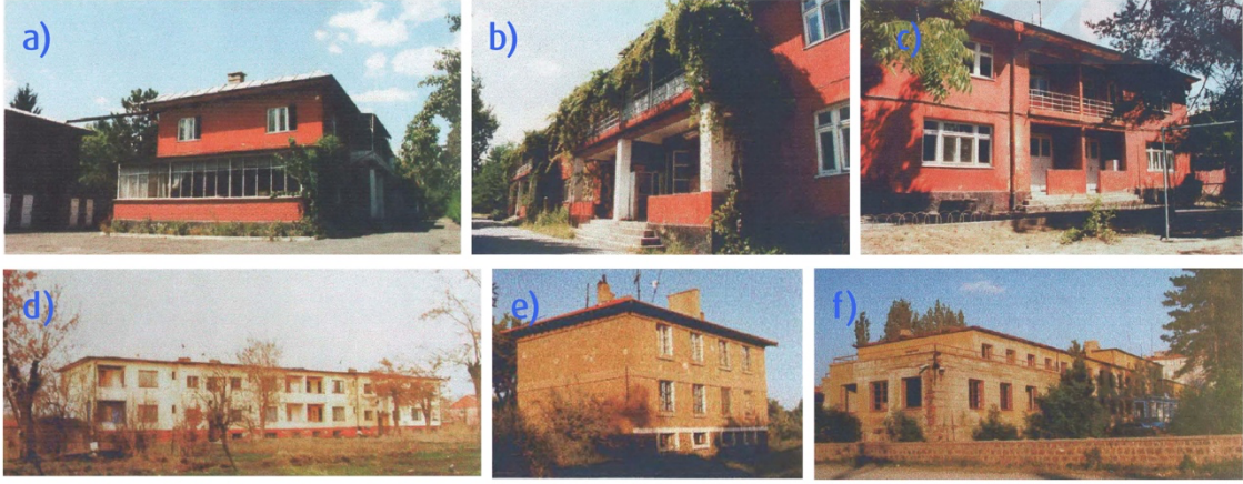
Şekil 2. Sümerbank Kayseri Bez Fabrikası Farklı Kullanıcı Gruplarına Ait Konut Tiplerine Konut Ait Cephe Görünüşleri. a) Tip 1A – Genel Müdür Konutu, b) Tip 1 – Müdür Yardımcısı ve Bölüm Müdürü Konutu, c) Tip 2 – İdari Personel Konutu, d) Tip 3 – İşçi Konutu, e) Tip 4 – Memur ve Ustabaşı Konutu, f) Tip 5 – Bekar İşçi Konutu (Asiliskender, 2002, s. 80-90).
