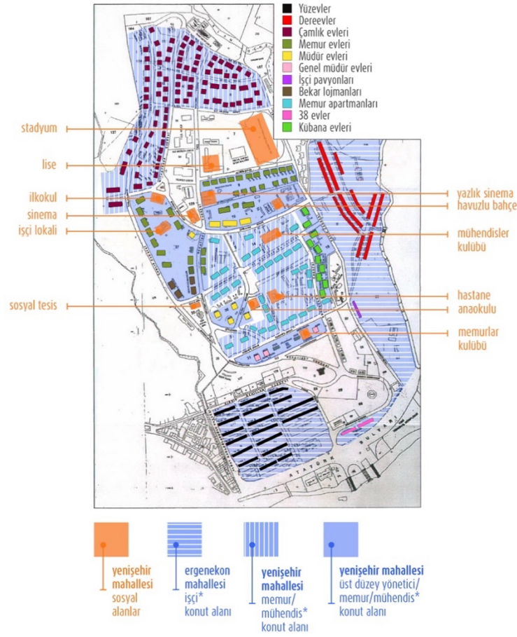
Şekil 4. Karabük Demir-Çelik fabrikası Planı ve Fonksiyonel Yapı Gruplaşması (Öktem, 2004, s. 88; yazar tarafından yeniden düzenlenmiştir)
