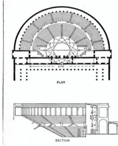
Fig. 24: Vitruvius'a göre Roma Tiyatro Planı (Fişenk-Satıcı 2021, 129)
